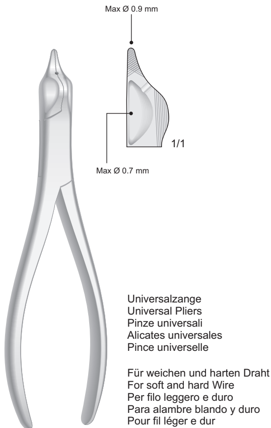
WALDSACHS DP-84 150 mm
